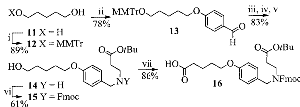
Scheme 2. Synthesis of the linker 16 : i) MMTrCl, Py; ii) 4-hydroxybenzaldehyde, DEAD, \text{Ph}_3\text{P} , THF; iii) \text{H}-\beta -Ala- O t Bu-HCl, DIPEA, \text{Na}_2\text{SO}_4 , \text{CH}_2\text{Cl}_2 ; iv) \text{NaBH}_3\text{CN} , AcOH, MeOH; v) AcOH; vi) FmocCl, DIPEA, dioxane; vii) \text{CrO}_3 , \text{H}_2\text{O} , \text{H}_2\text{SO}_4 , acetone
